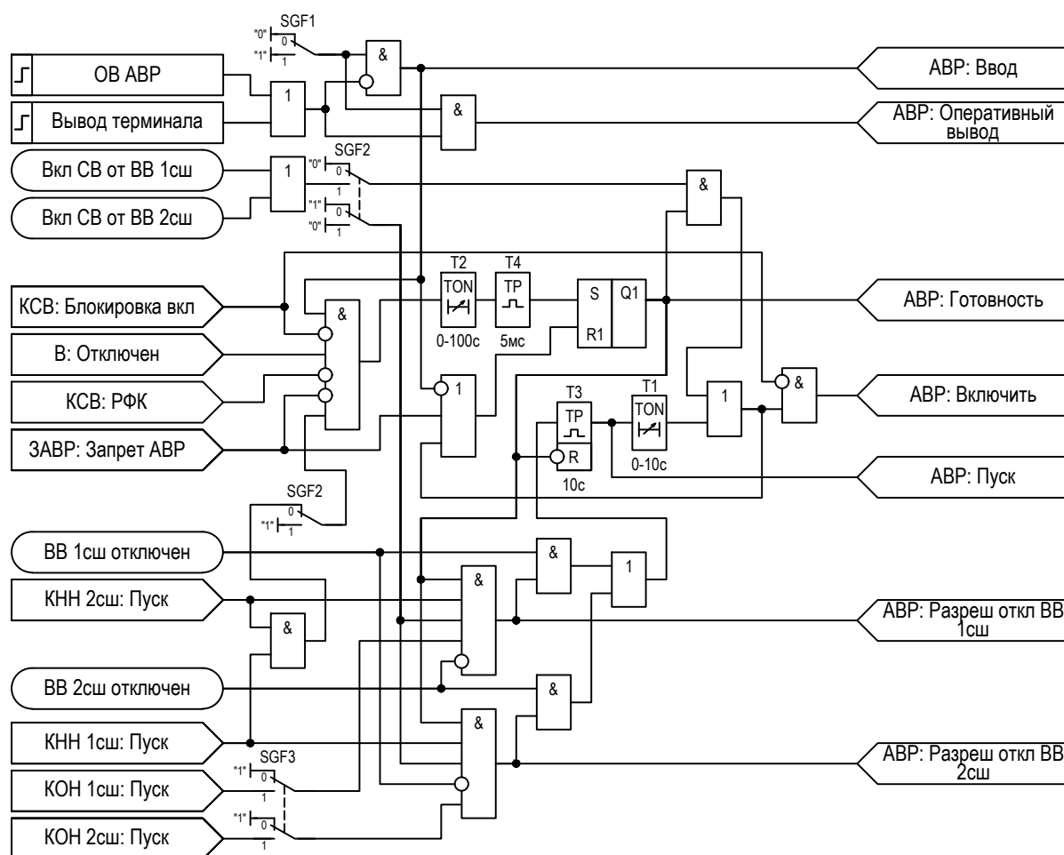
Рисунок 2.39 – Функциональная схема «АВР»
