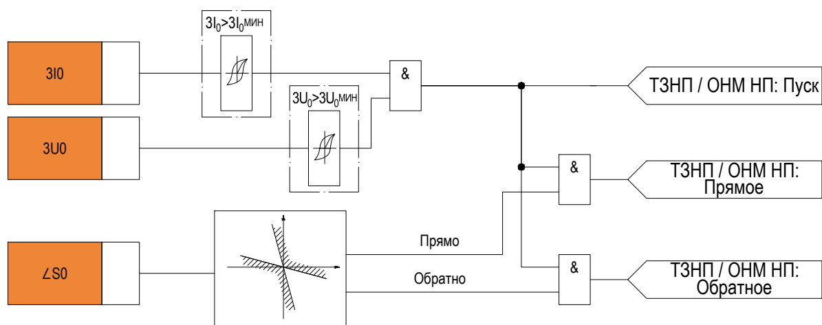
Рисунок 2.29 – Функциональная схема «ОНМ НП»
