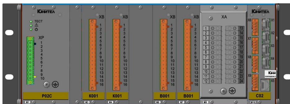
Рисунок 1.1 – Вид устройства «ЮНИТ-М314-СВ» с размещением модулей по слотам
